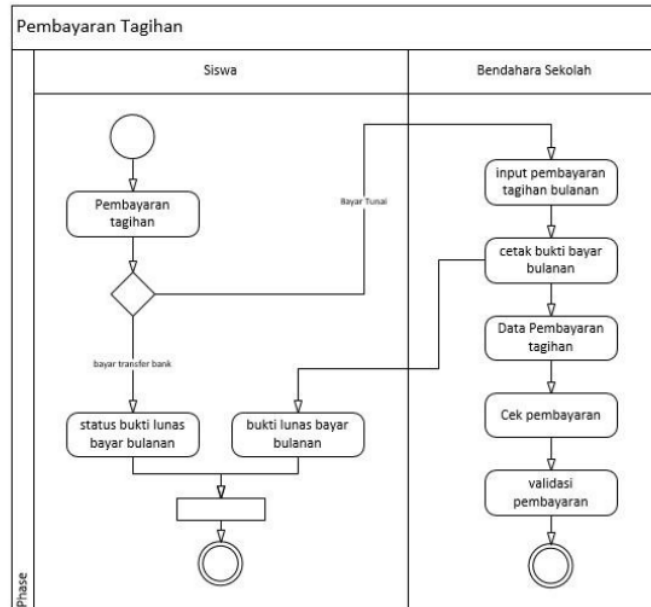
Gambar 5. Aktifitas Pembayaran tagihan
