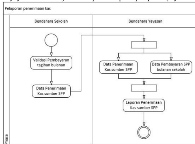
Gambar 6. Aktifitas penerimaan kas
