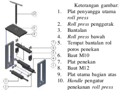
Gambar 7. Proses Perakitan Roll Press
