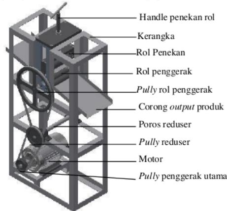
Gambar 4. Desain Roll Press
