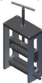
Gambar 6 Roll Press
