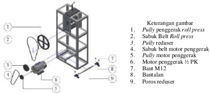
Gambar 8. Proses Pemasangan Komponen Sistem Penggerak
