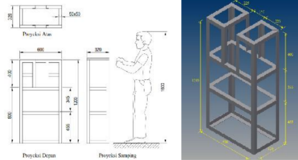
Gambar 5. Kerangka Roll Press
