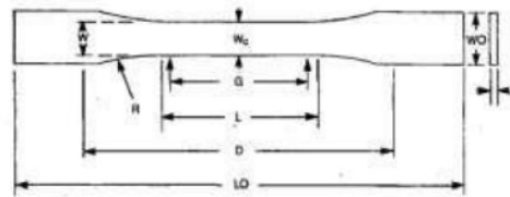
Gambar 2 Bentuk Spesimen Uji Tarik [21]
