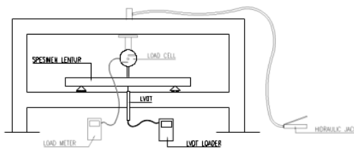
Gambar 3 Sketsa Setup Pengujian Lentur
