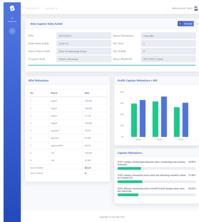
Gambar 14. Antarmuka hasil capaian penilaian peserta kelas
