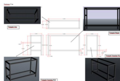
Gambar 1 Desain Rangka Pengering Menjes
