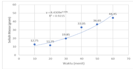
Gambar 4 Grafik Perubahan Massa Menjes Terhadap Lama Pemanasan Pada T = 40° C
