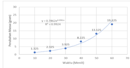
Gambar 5 Grafik Perubahan Massa Menjes Terhadap Lama Pemanasan Pada T = 50° C
