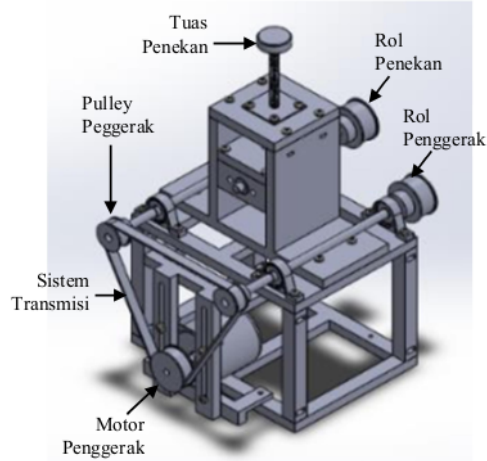
Gambar 5. Prototipe Mesin Rol Pelat
