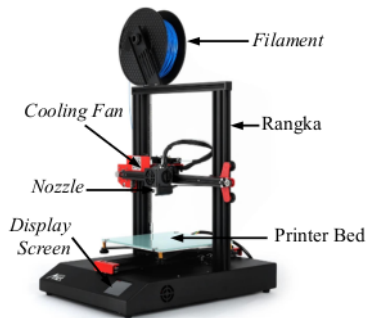
Gambar 4. Mesin Cetak 3D.
