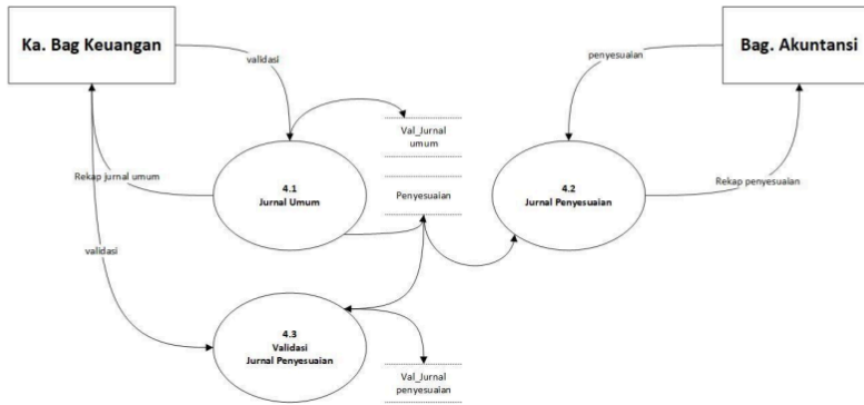
Gambar 4. Diagram Konteks Desain Sistem Informasi Akuntansi yang Diusulkan Level 1-4
