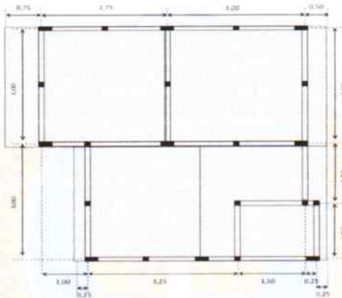
Gambar 3 Denah Rumah Tipe 38
